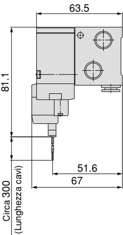
Connettore ad innesto L (L)
