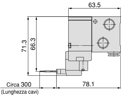
Connettore ad innesto M (M)
