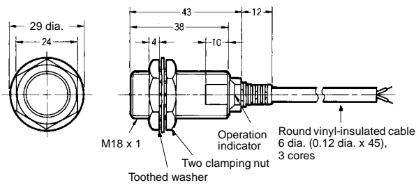
Fig. 7 : E2EG-X10Cj /Bj
