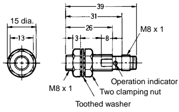
Fig. 17 : E2EG-X1R5C1-M3/B1-M3
