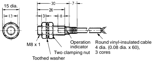
Fig. 1 : E2EG-X1R5Cj /Bj
