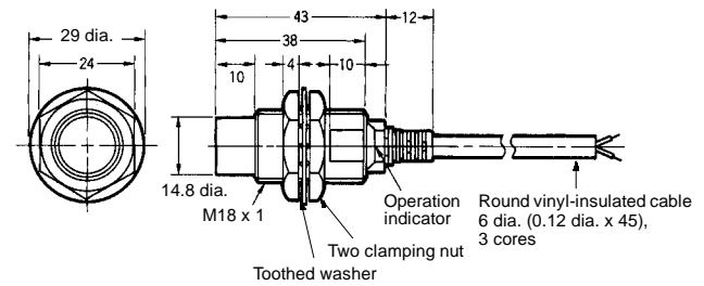
Fig. 8 : E2EG-X18MCj /Bj
