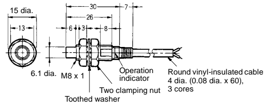
Fig. 2 : E2EG-X2MCj /Bj
