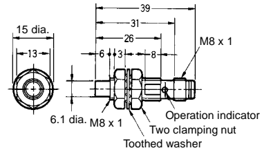
Fig. 18 : E2EG-X2MC1-M3/B1-M3
