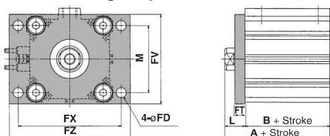
Rod side flange style: CQ2F/CDQ2F
